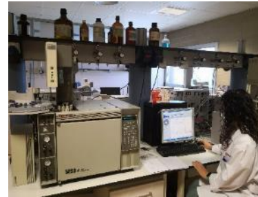
Cromatografía
